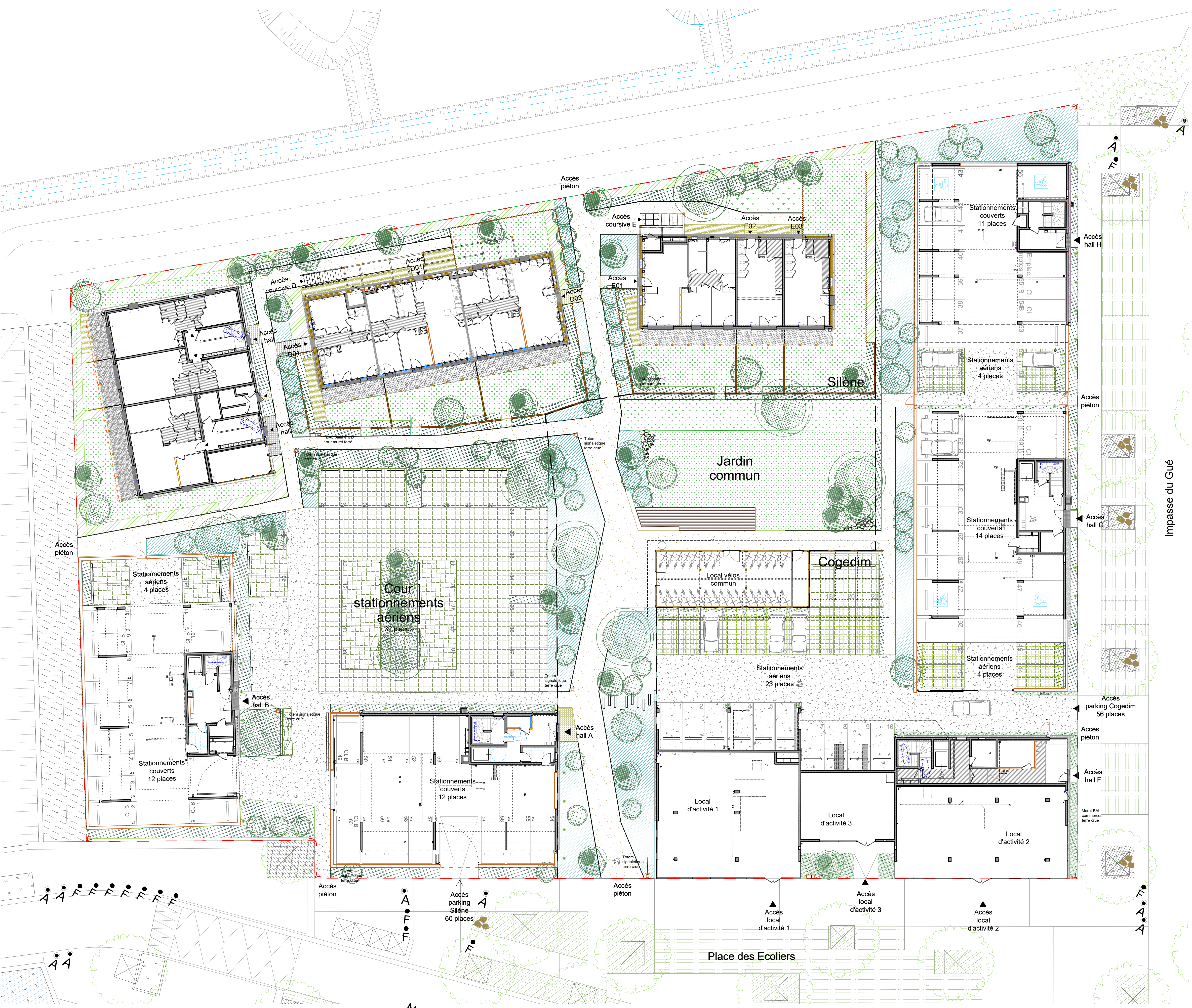
Plan de rez-de-chaussée 1/200e
