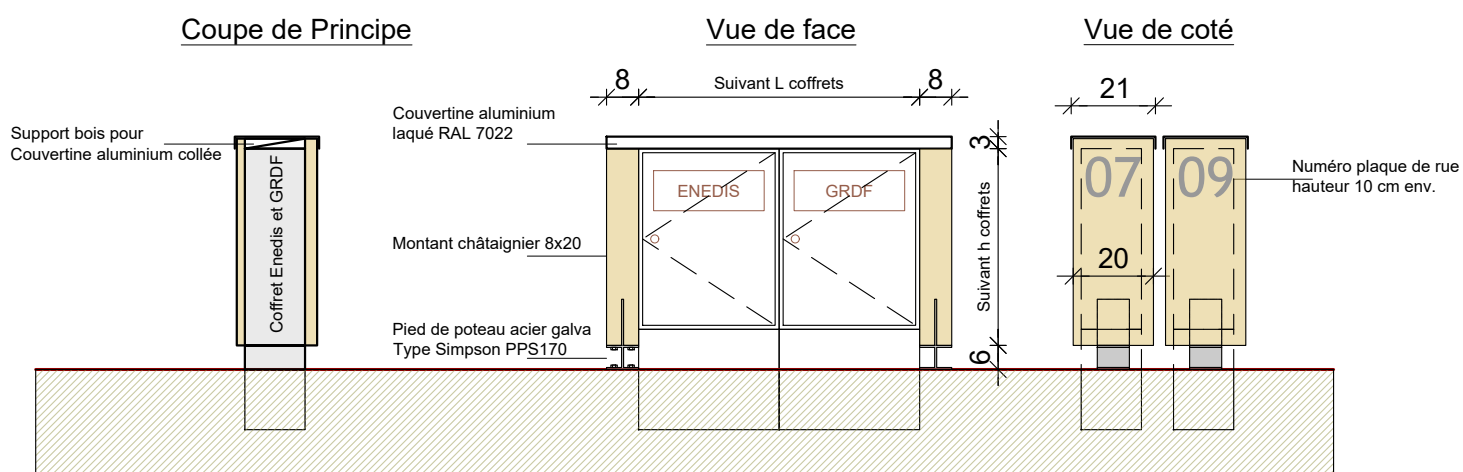
Plans de principe à ajuster suivant dimensions et implantations des coffrets
